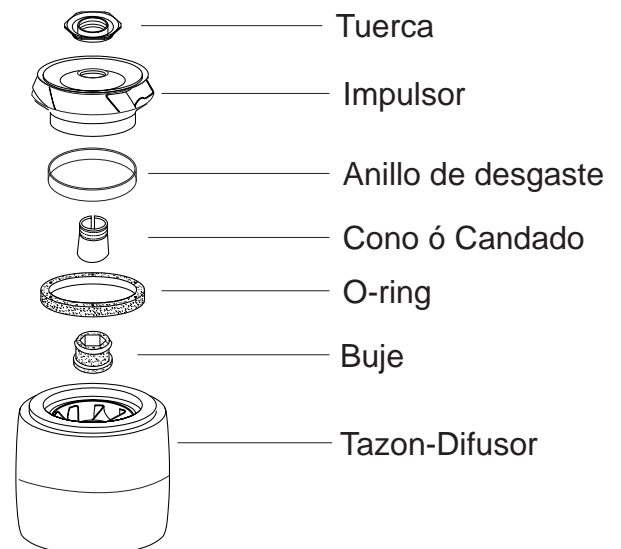
Figura 3: Etapa completa de bomba de 6"
