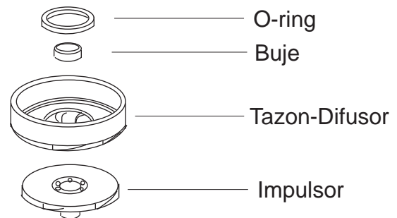
Figura 2: Etapa completa de bomba de 4"
